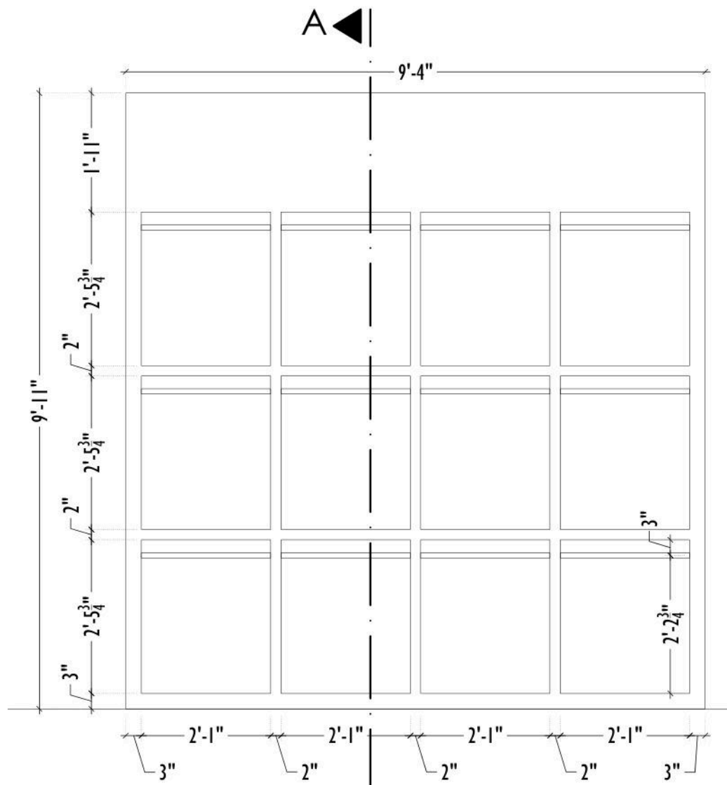
ELEVATION A-A'
